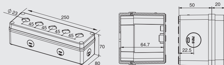
型号 ( Model ) : DS-AG-0825-K5Y 尺寸 ( Size ) : 80X250X70mm
