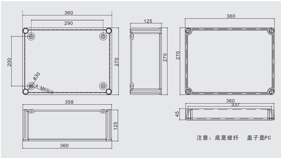
Dimension(允许误差 ± 1mm)
