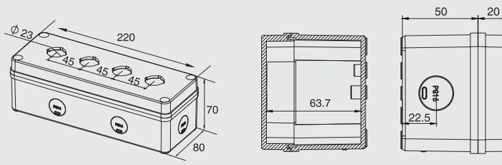
型号 ( Model ) : DS-AG-0822-K4Y 尺寸 ( Size ) : 80X220X70mm
