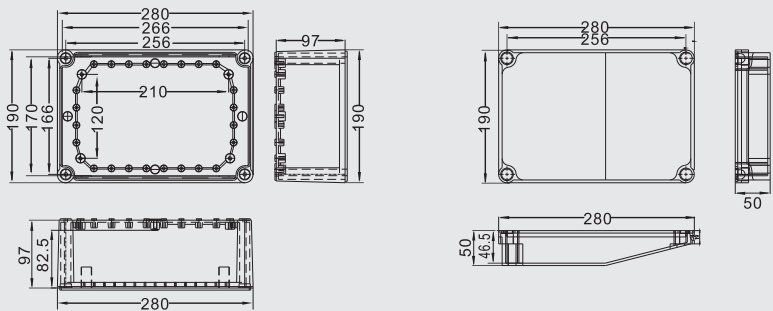
Dimension(允许误差 ± 1mm)
