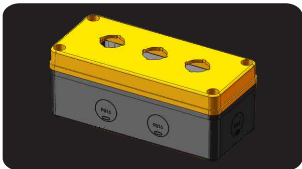
型号 ( Model ) : DS-AG-0818-K3Y 尺寸 ( Size ) : 80X180X70mm
