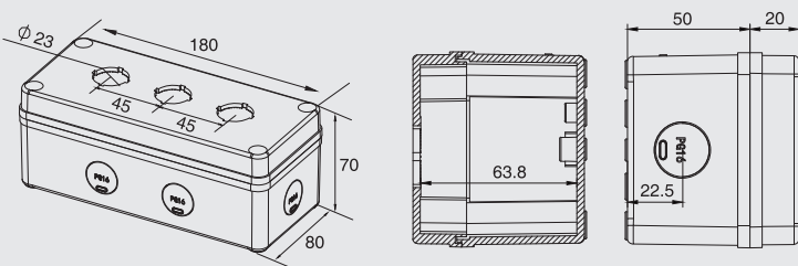
型号 ( Model ) : DS-AG-0818-K3Y 尺寸 ( Size ) : 80X180X70mm
