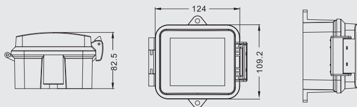
型号(Model): DST-01 尺寸(Size): 124×110×82mm
