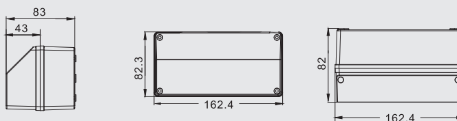
型号(Model): DST-04 尺寸(Size): 160×82×82mm
