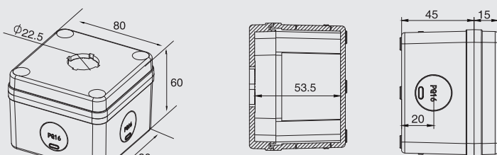
型号 ( Model ) : DS-AG-0808-K1Y 尺寸 ( Size ) : 80X80X60mm
