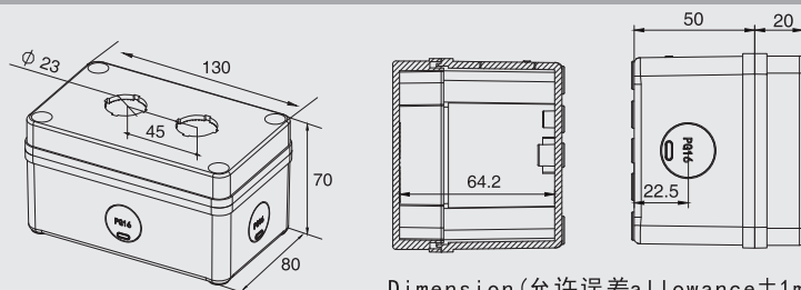
型号 ( Model ) : DS-AG-0813-K2Y 尺寸 ( Size ) : 80X130X70mm
