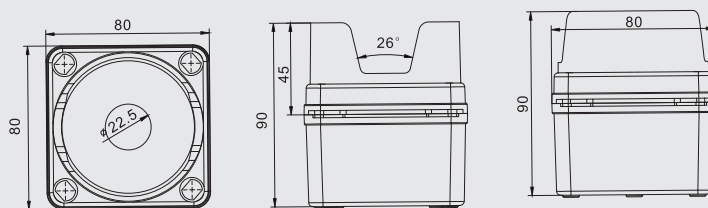
型号(Model): DST-02 尺寸(Size): 80×80×90mm
