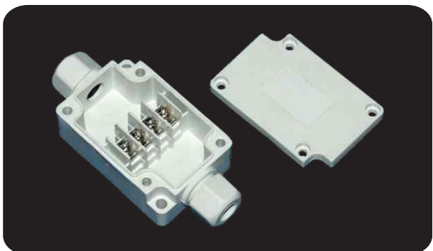
型号 (Model) : PBT-4P 尺寸 (Size) : 40×60×24mm
