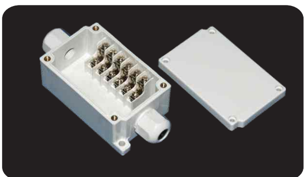
型号 (Model) : DS-MTB-6P 尺寸 (Size) : 55×125×40mm
