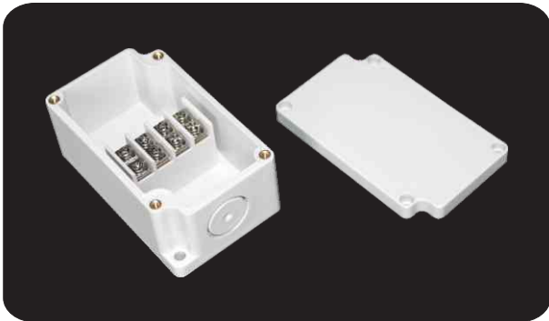
型号 (Model) : DS-4P-M 尺寸 (Size) : 55×91×43mm
