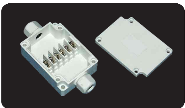
型号 (Model) : PBT-6P 尺寸 (Size) : 50×70×24mm
