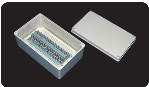
型号 (Model) : DS-AG-40P-S 尺寸 (Size) : 150×250×100mm
