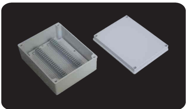
型号 (Model) : DS-AG-40P-M 尺寸 (Size) : 200×250×100mm
