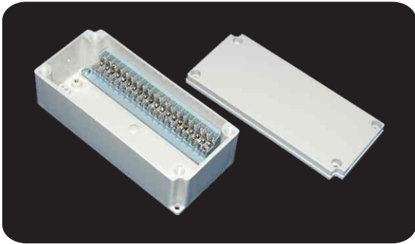
型号 (Model) : DS-PG-20P-S 尺寸 (Size) : 100×223×75mm
