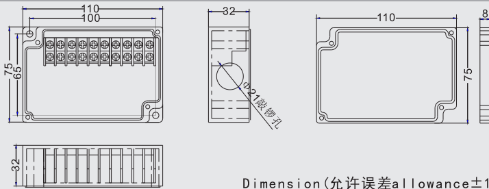
型号 (Model) : DS-PG-10P 尺寸 (Size) : 75×110×40mm
