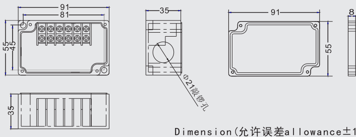
型号 (Model) : DS-6P-K 尺寸 (Size) : 55×91×43mm
