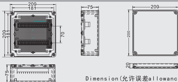
型号 (Model) : DS-AG-30P-M 尺寸 (Size) : 200×200×95mm
