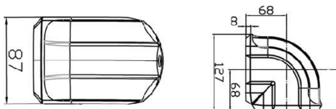
品名:转角 订货号:60-95-310 重量:0.7kg 材料:压铸铝合金
