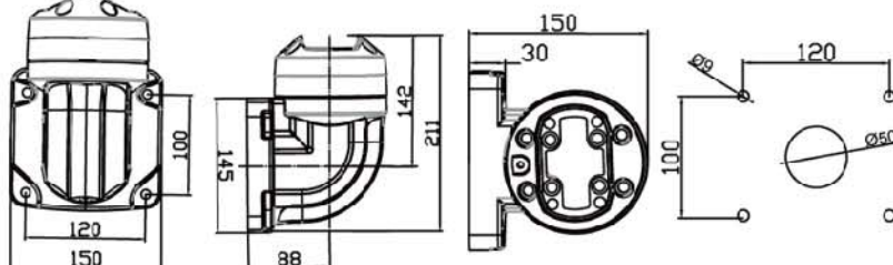
品名:垂直墙座 订货号:60-95-370 重量:2.7kg 材料:压铸铝合金 可旋转320°
