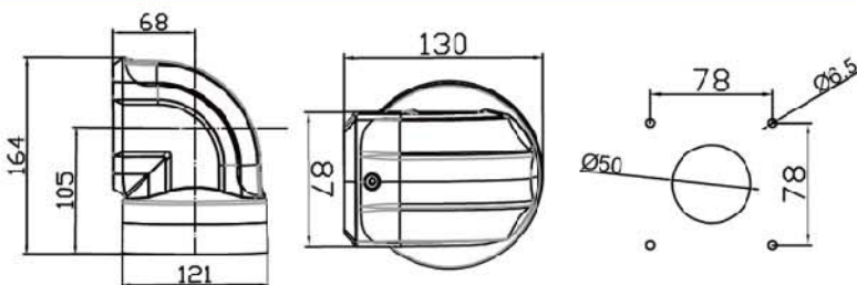
品名:90° 箱体连接器 订货号:60-95-350 重量:1.5kg 材料:压铸铝合金 可旋转320°
