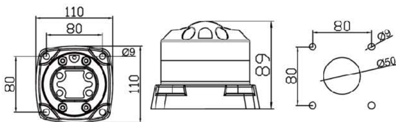
品名:底座 订货号:50-65-280 重量:0.9kg 材料:压铸铝合金 可旋转320°
