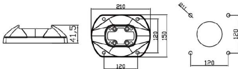
品名:固定底座 订货号:75-110-540 重量:0.9kg 材料:压铸铝合金
