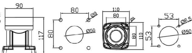
品名:可旋转箱底座 订货号:50-65-4900 重量:0.8kg 材料:压铸铝合金 可旋转320°
