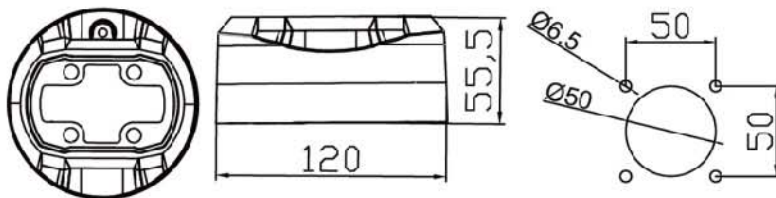
品名:箱体连接器 订货号:60-95-3090 重量:0.9kg 材料:压铸铝合金 可旋转320°
