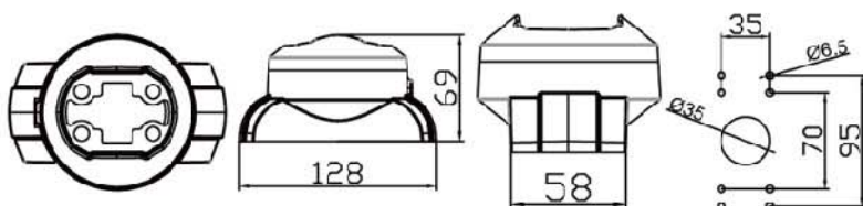
品名:窄边箱体连接器 订货号:50-65-2091 重量:0.5kg 材料:压铸铝合金
