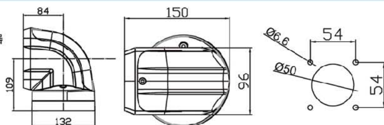
品名:90°箱体连接器 订货号:75-110-550 重量:1.8kg 材料:压铸铝合金 可旋转320°
