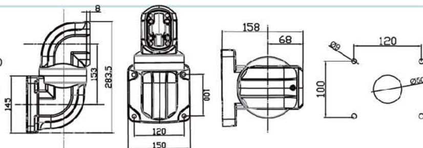
品名:水平墙座 订货号:60-95-360 重量:2.9kg 材料:压铸铝合金 可旋转320°
