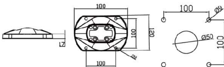
品名:固定底座 订货号:60-95-340 重量:0.6kg 材料:压铸铝合金
