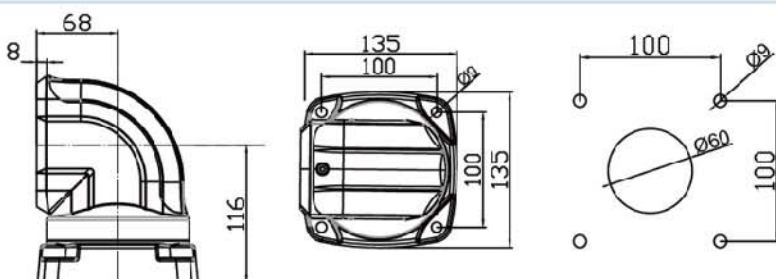
品名:顶座 订货号:60-95-320 重量:1.8kg 材料:压铸铝合金 可旋转320°
