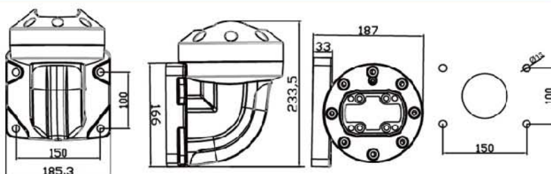
品名:垂直墙座 订货号:75-110-570 重量:5.1kg 材料:压铸铝合金 可旋转320°
